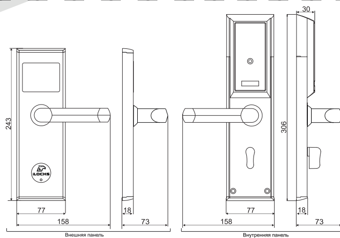
Рисунок №1 – Структурная схема (спецификация) замков и габариты замков типа iLOCKS IS8005A3B3
