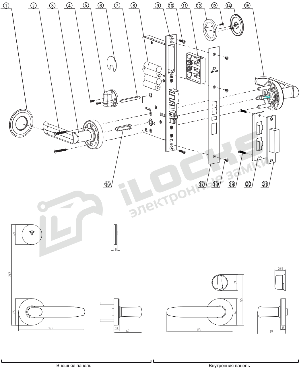
Рисунок №1 – Структурная схема (спецификация) замков типа iLOCKS IS190 433+BLE
