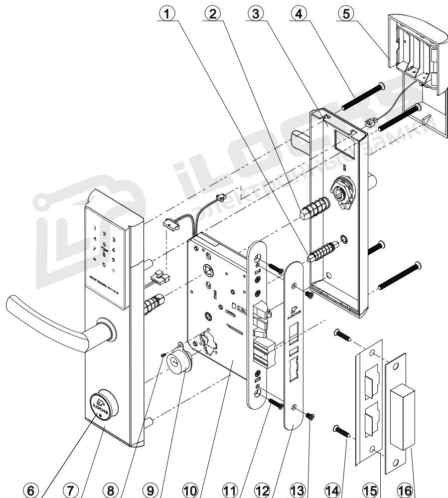
Рисунок №1 – Структурная схема (спецификация) замков типа IS8005AB3-BL
