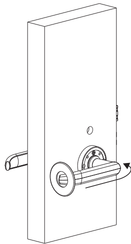
Рисунок №5.2 – Установка декоративной накладки задней (внутренней) ручки
