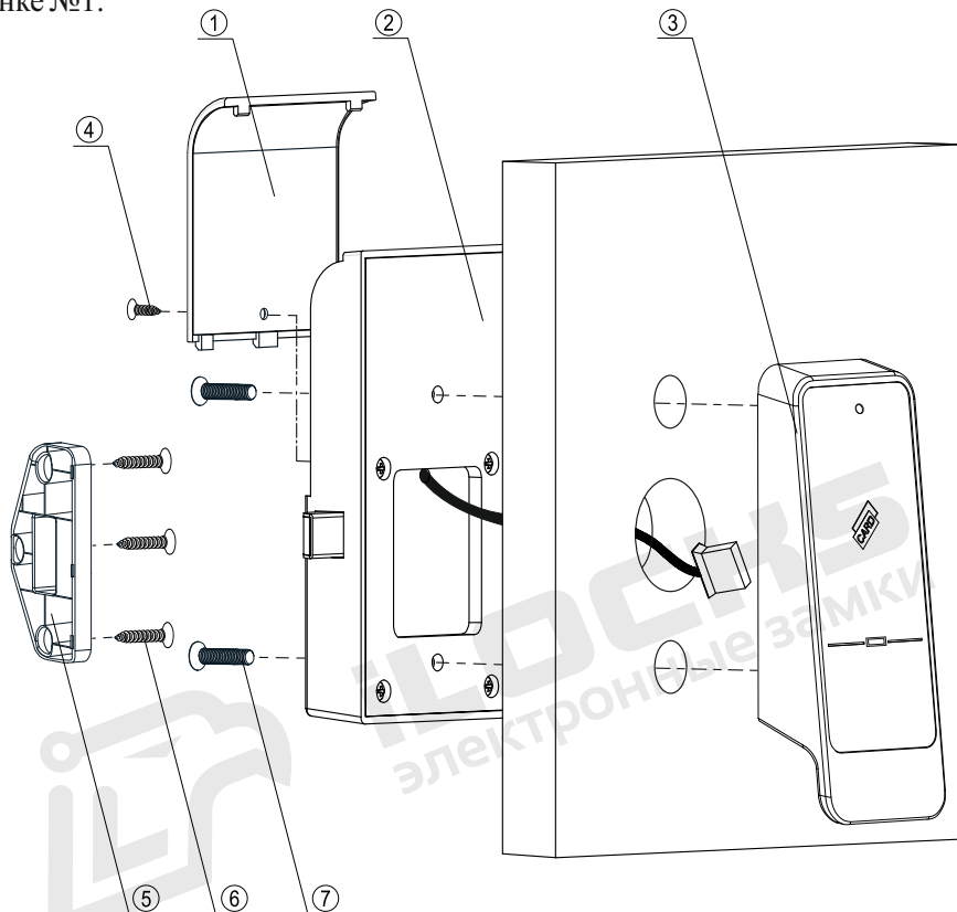
Рисунок №1 – Структурная схема (спецификация) замка типа IS0860-MF
