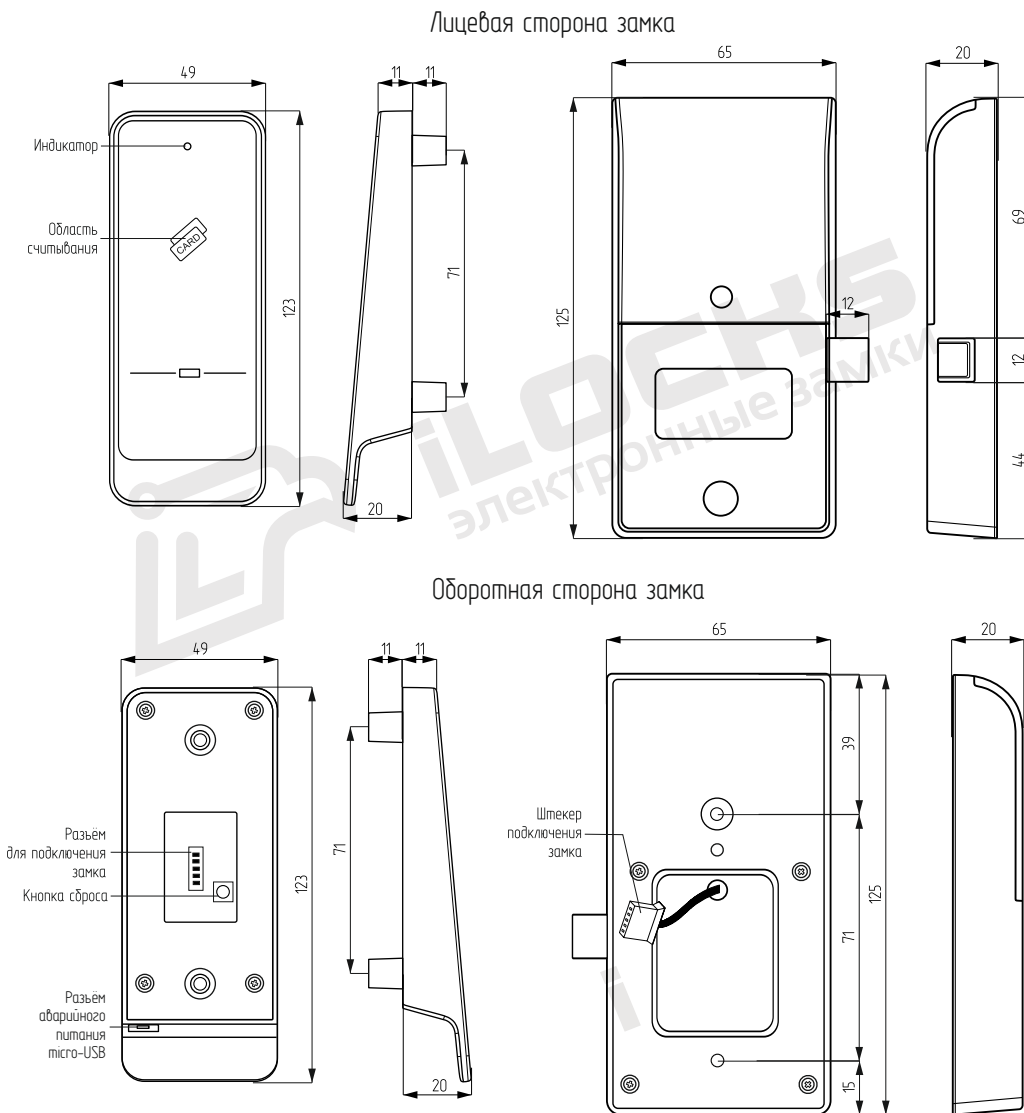
Рисунок №2 – Габаритные характеристики замка типа IS0860-MF
